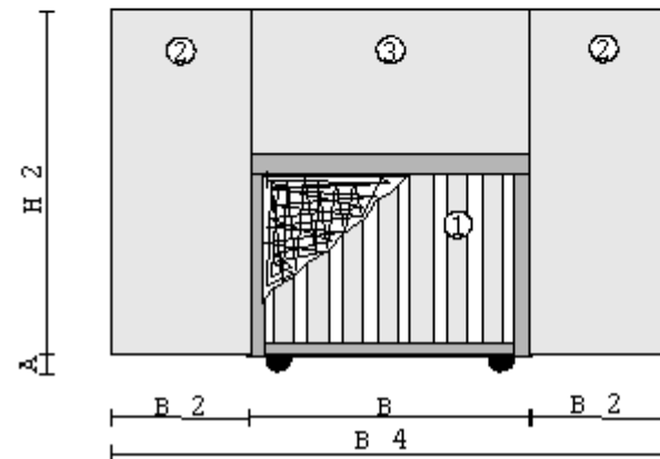
Gerät mit Filtermatte, vorgeschaleteten Prallblech- Labyrinth-Filtern (1) und Mobil-Set bestehend aus schwenk- und arretierbaren Seitenteilen (2) sowie Abweisblech (3)
